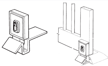
MEA1 Dispositif pour ouverture à 360°
