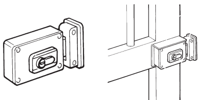
MEA2 Débrayage à serrure
